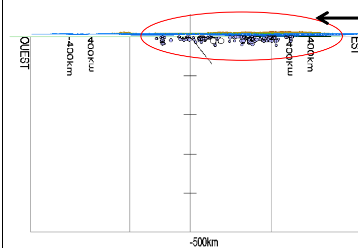
Bloc 3D au niveau de l'Islande avec affichage de la distribution des foyers sismiques selon la profondeur
