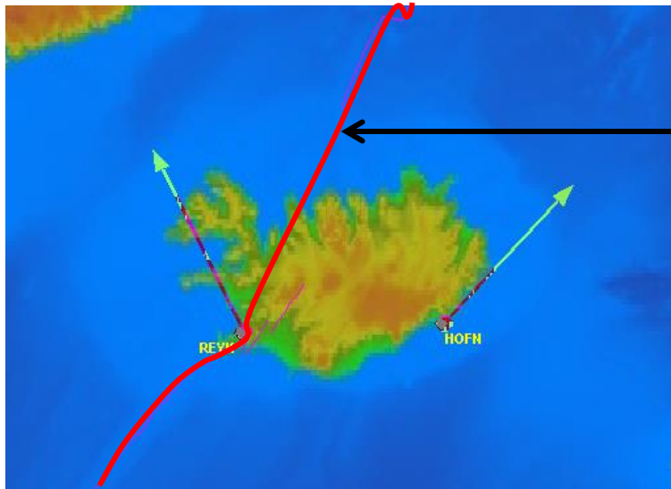
Déplacement relatif des balises GPS (station REYK et HOFN) en Islande
